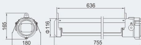
HRY92-LED20□□ HRY92-LED40□□
