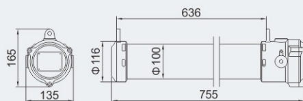
HRY92-LED20□□ HRY92-LED40□□
