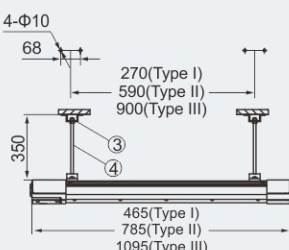
G: pendant pole type
