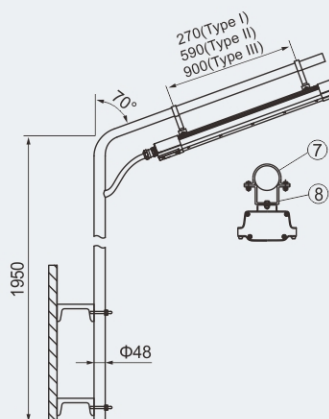
W: bend pole type
